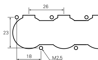
〈取付穴寸法〉
