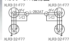
R300-CN結線図
