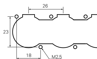
〈取付穴寸法〉
