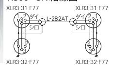
R300-CN結線図
