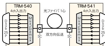
TRM-540/541 ブロック図
