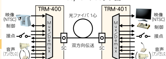
TRM-400/401ブロック図
