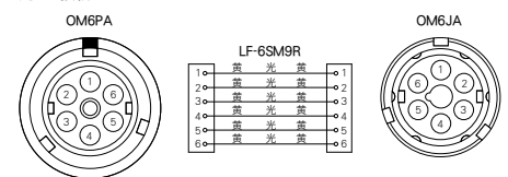
光6心接続ケーブル
