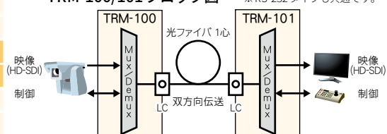
TRM-100/101ブロック図
