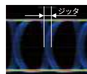
b) ジッタ=210psの波形
