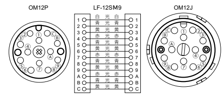
光12心接続ケーブル
