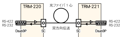
TRM-220/221 ブロック図
