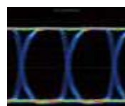
a) ジッタ=93psの波形
