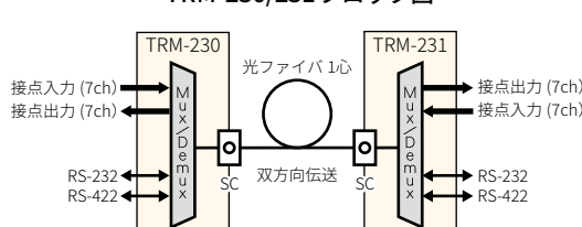
TRM-230/231ブロック図
