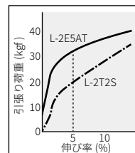
ケーブルの引張り荷重と伸び率
