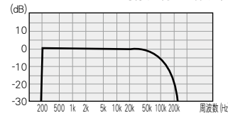
L-2B2AT 周波数特性 (長さ100m)
