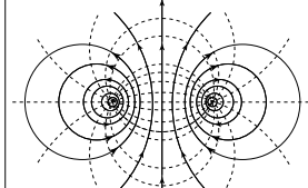
〈図2〉2心ケーブルに発生した磁界
