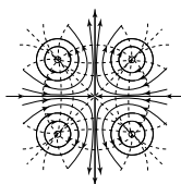
〈図1〉4心ケーブルに発生した磁界
