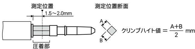
クリンプハイトの測定位置と算出方法
